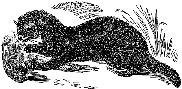
Polecat ( Mustela putorius ).
